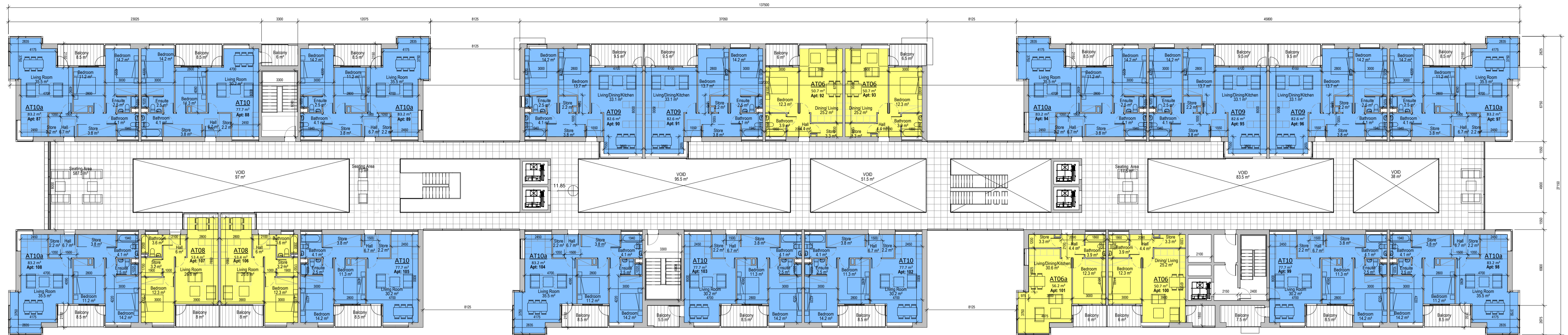
1 Block 01 - Level 04 1 : 200
